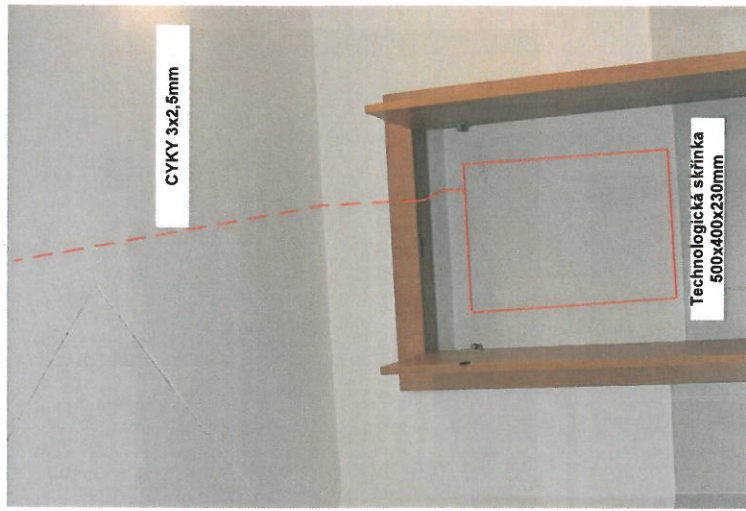
9. 2NP místnost 2.10 Umístění technologické skříňky ve falešné skřínce.
