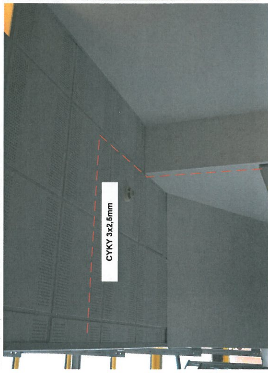
2. Instalace NN kabelu za sádrokartonovou stěnu následně přechod do podhledového prostoru nad kazetový strop. Kabel bude směřovat do místnosti WC č. 1.13
